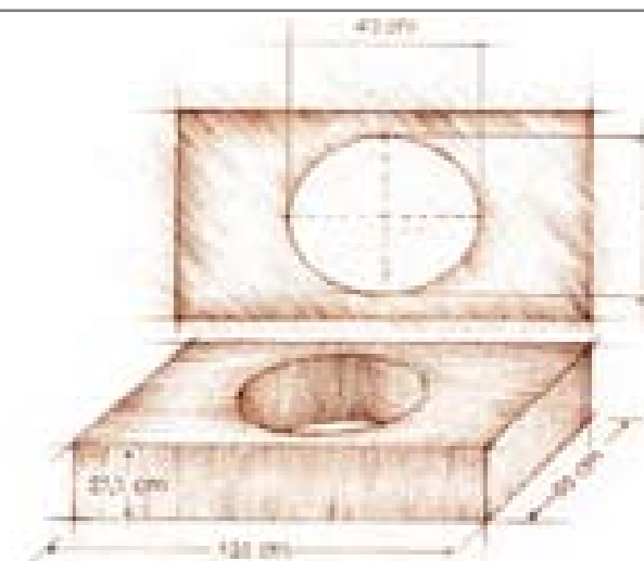
T2 - BASE IN LEGNO DA PIASTRELLARE (LEGNO MULTISTRATO DI CONIFERA, SPESSORE MM 15) 120X60X21,3 CON FORO OVALE 49X39
